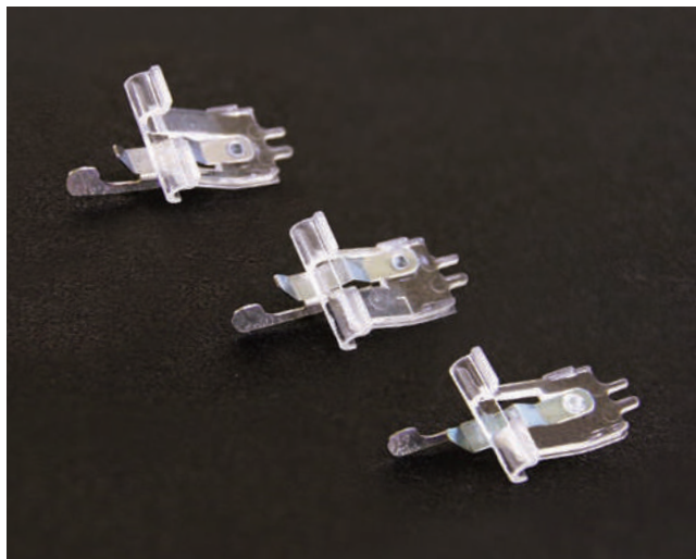
Inserti a canalina Part no. A-D2-01A (guida centrale) A-D2-02A (guida destra) A-D2-03A (guida sinistra)
