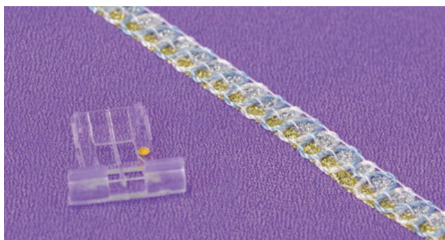
● Piedino cordoncino 2.5mm x 2 scanalature (giallo) Part no. A-D2-05A
